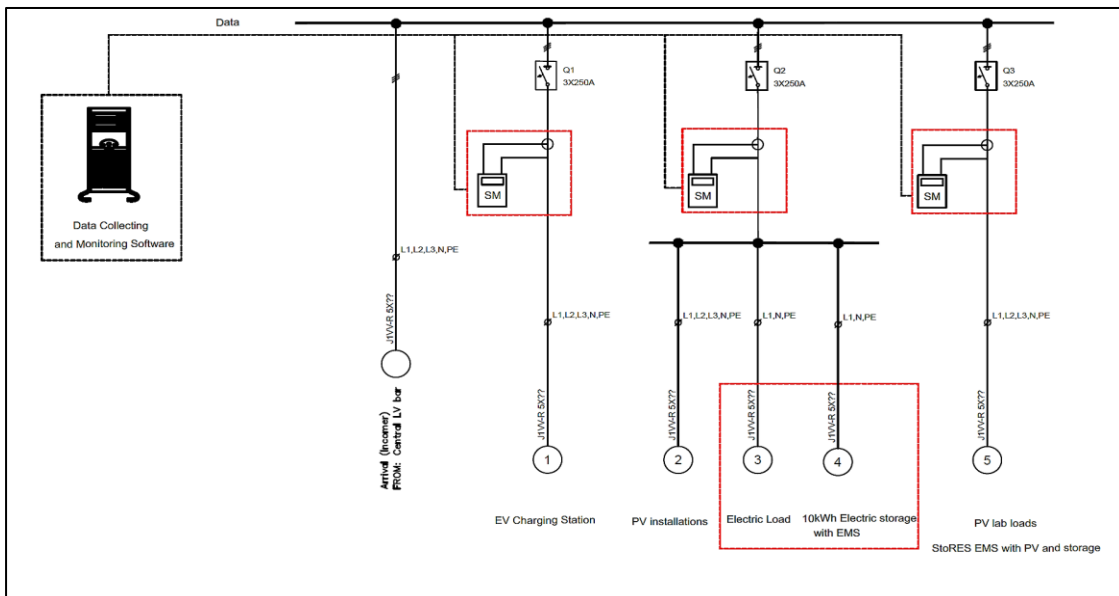
Schéma unifilaire du site pilote "nanogrid" de Chypre
